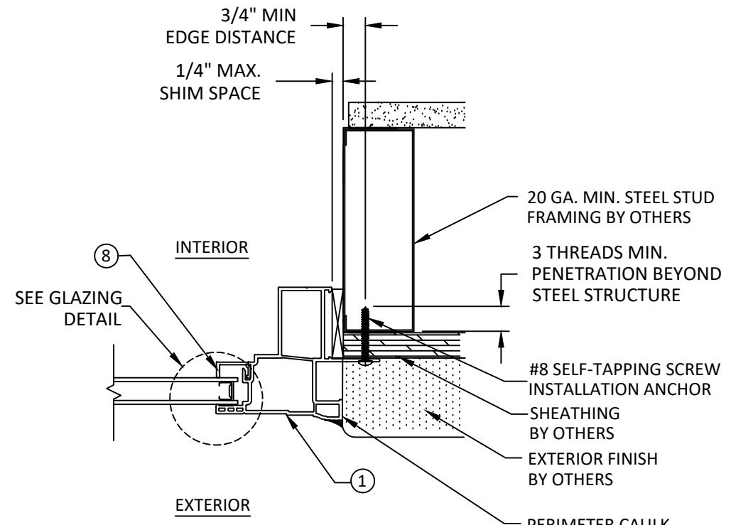
B 2 HORIZONTAL SECTION JAMB - STEEL STUD FRAME NAIL FIN
